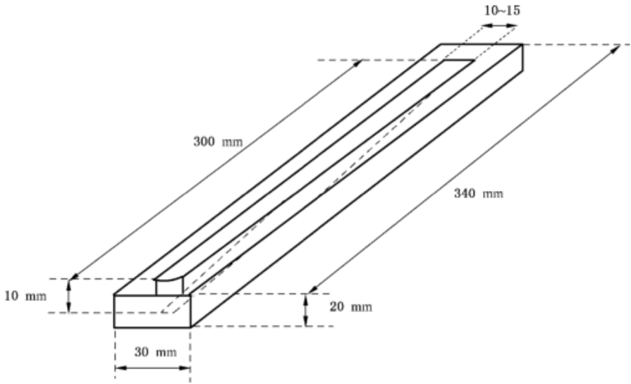
图 1 楔形凹槽
