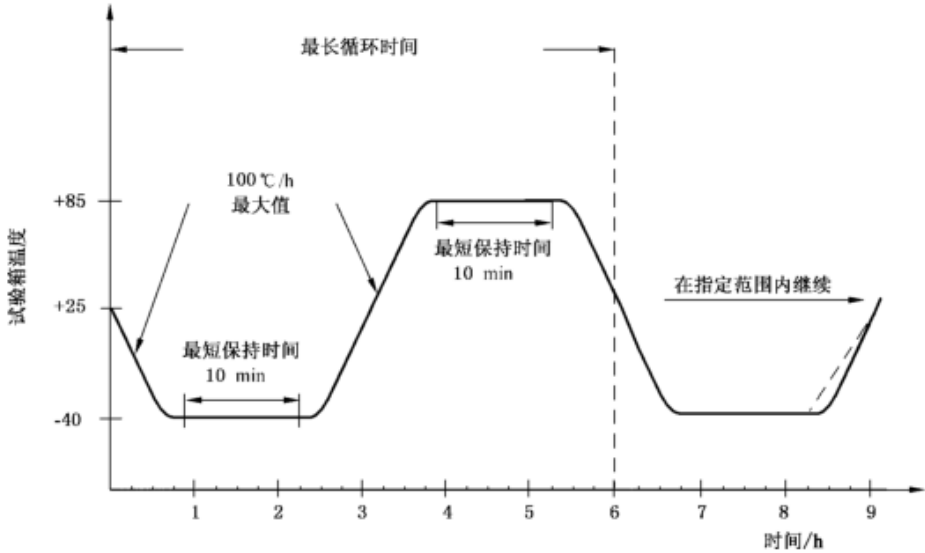
图 2 热循环试验
