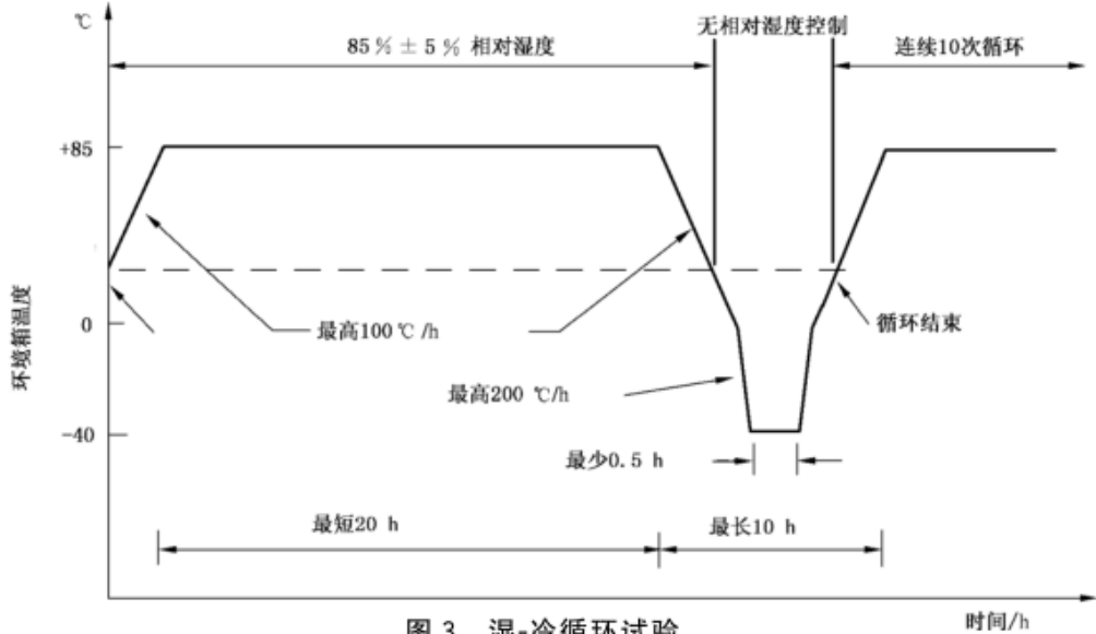
图 3 湿-冷循环试验
